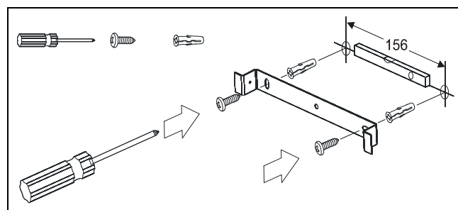
Abb. 2: Bohrmaße
