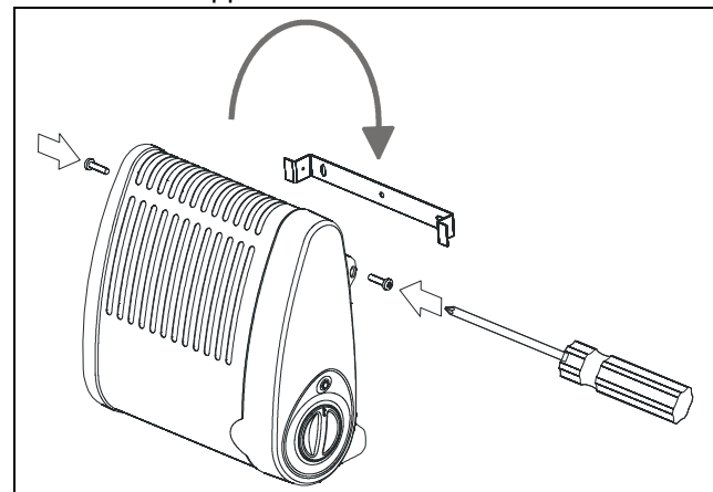
Abb. 3: Opérations de montage
