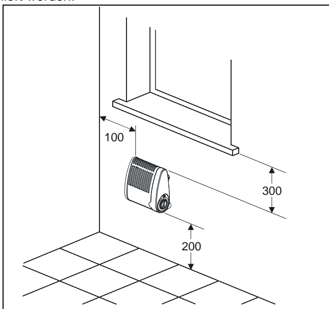
Abb. 1: Mindestabstände
