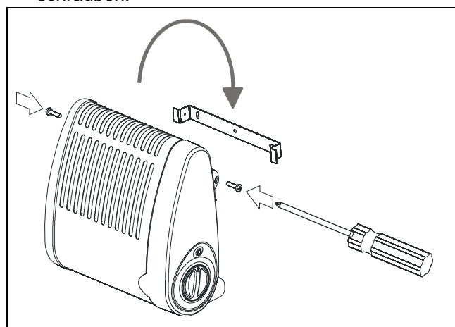
Abb. 3: Gerätemontage
