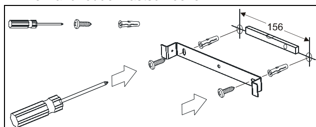
Abb.2: Dimensions voor gaten
