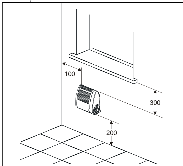
Abb. 1: Les dégagements minimaux
