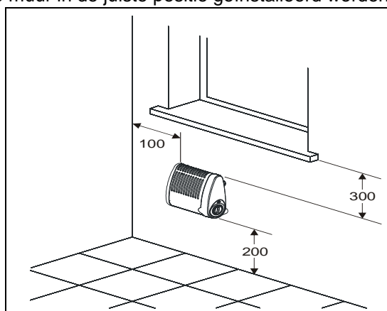
Abb.1: Minimumafstanden
