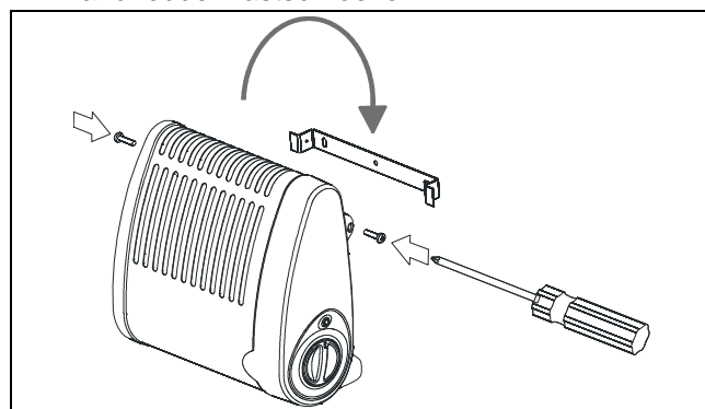
Abb. 3: Montage
